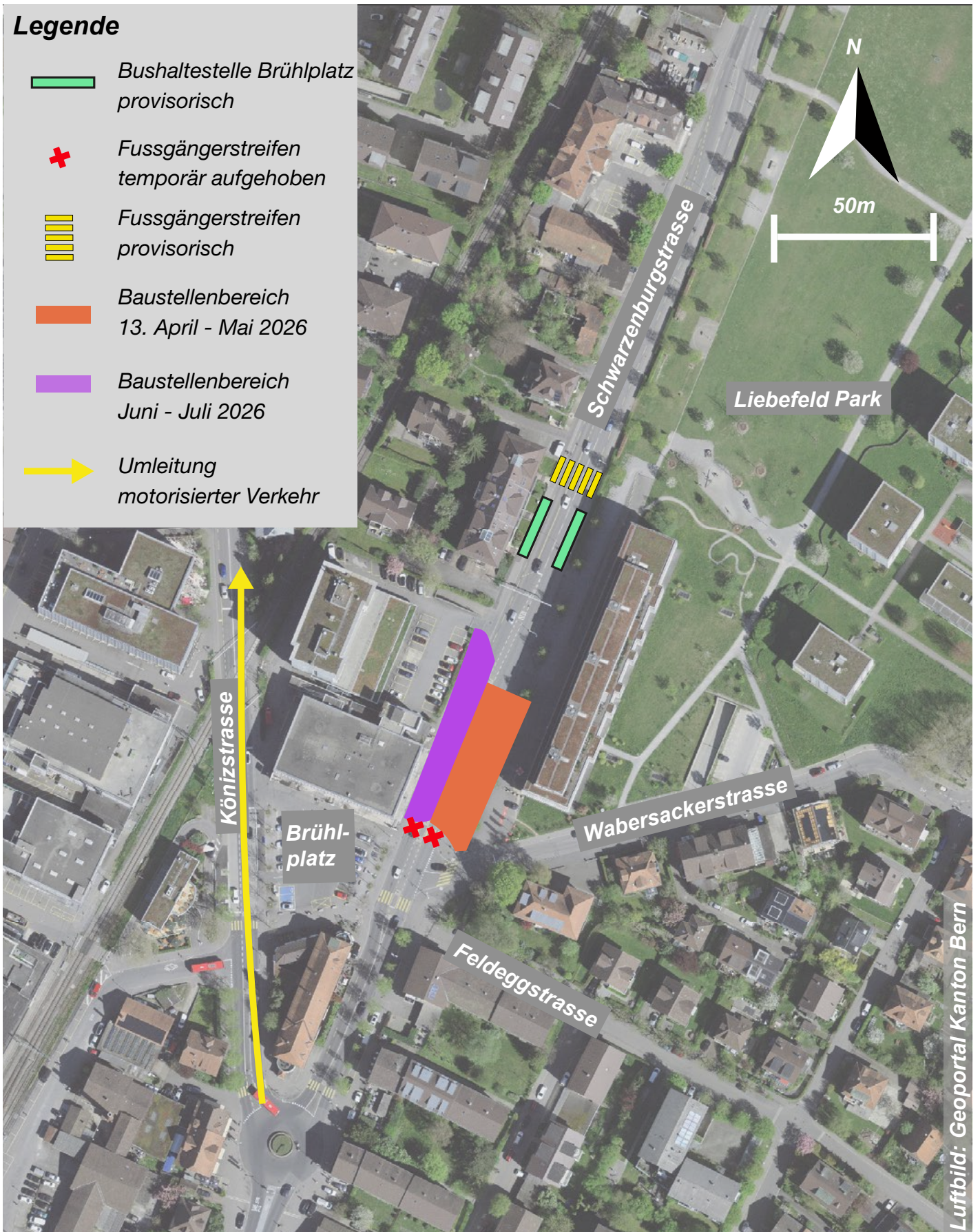
Umstellung Buslinie 10 auf Doppelgelenktrolleybusse: Übersicht Bauarbeiten Haltestelle Brühlplatz.
