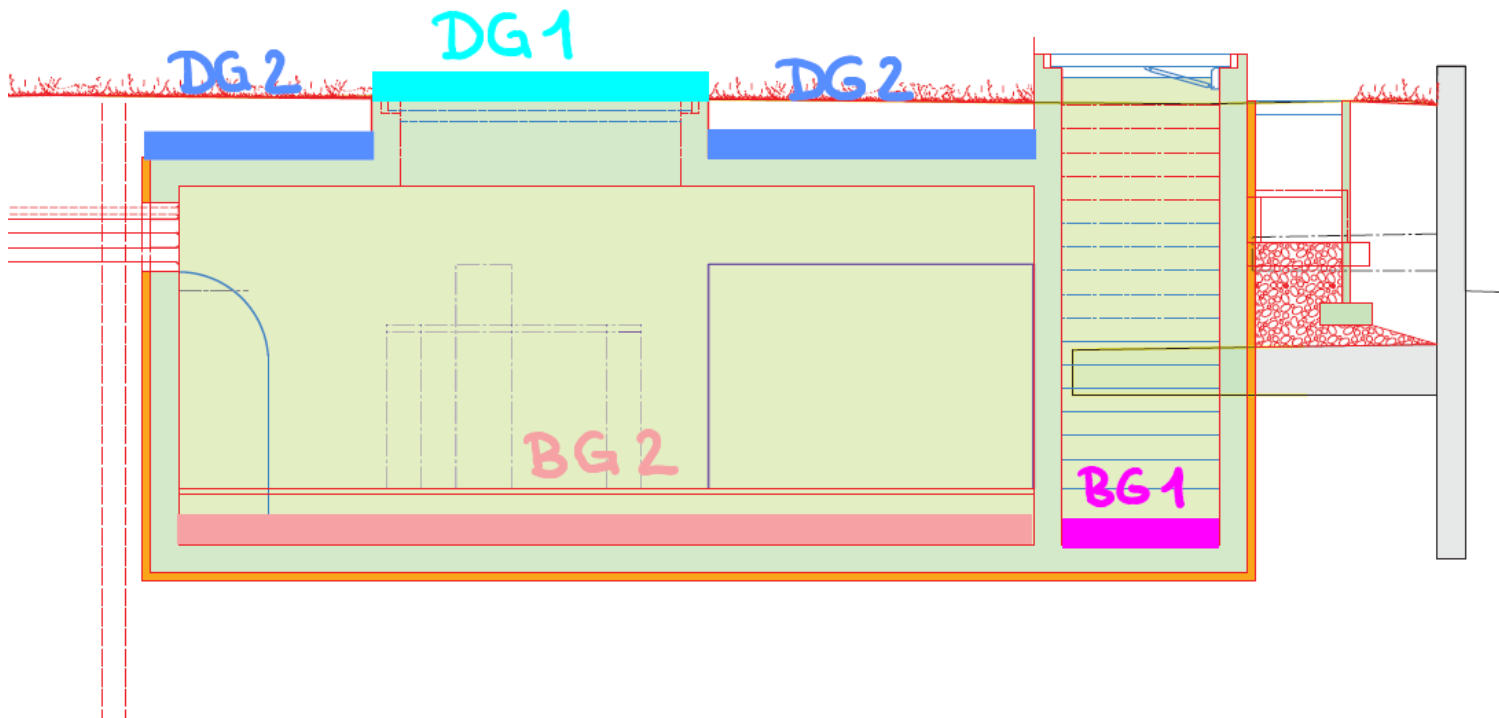
Abbildung 3: Nutzlasten und Auflasten Liebefeldpark
