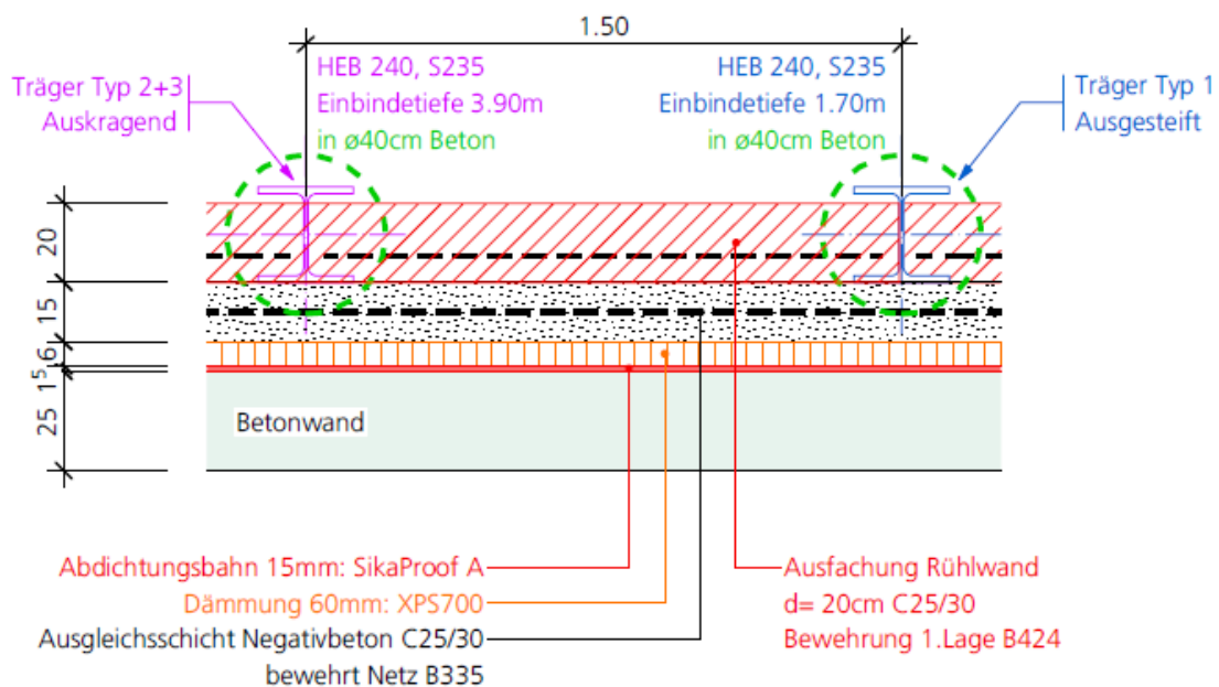
Abbildung 2: Schemaschnitt Rühlwand
